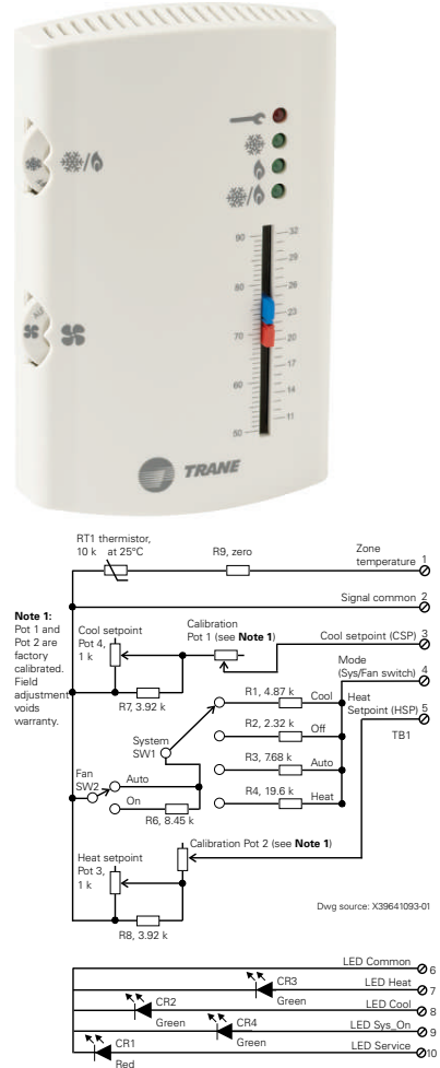
Figure 62. BAYSENS110*/ASYSTAT110*
