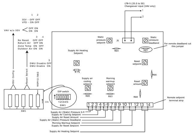
Figure 127. RTAM module
