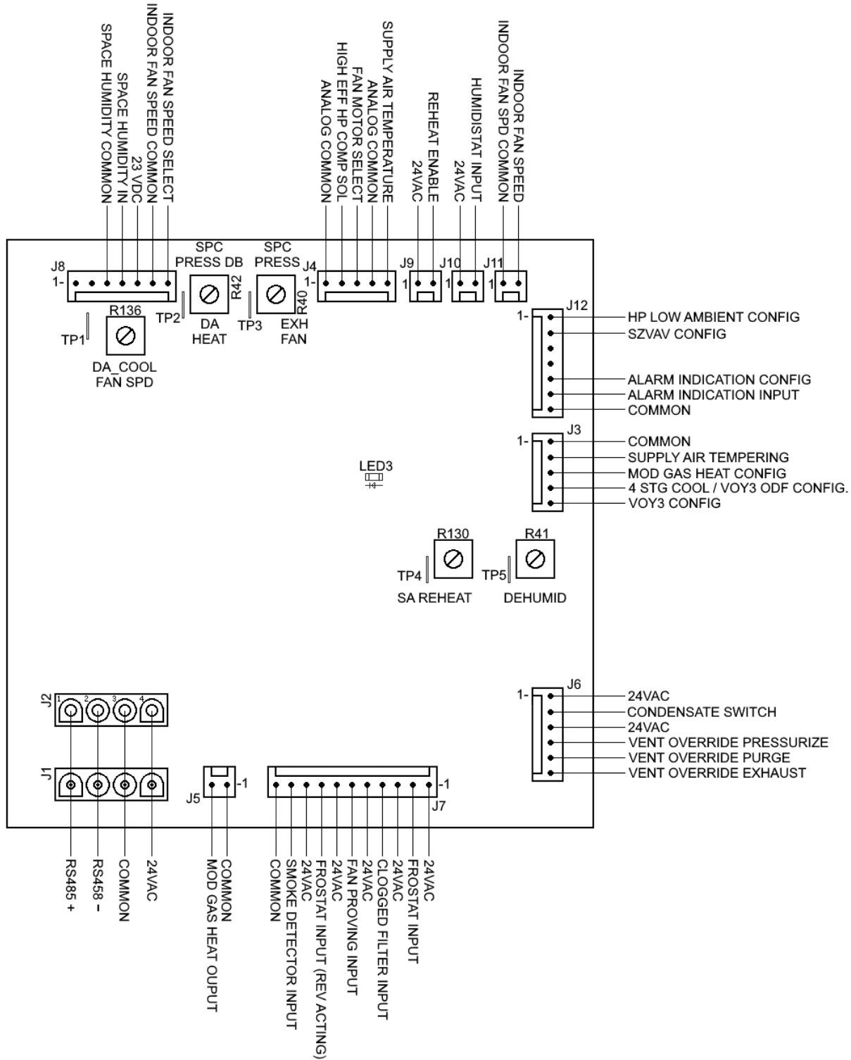
Figure 27. ReliaTel™ option module (RTOM)
